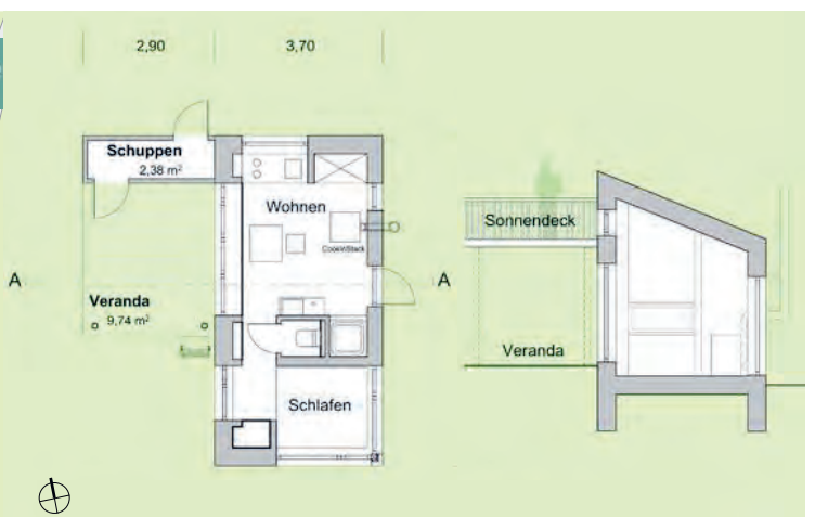
Haus Warumnicht – Grundriss EG, Schnitt A-A, ohne Maßstab, Quelle: © agmm Architekten + Stadtplaner, München
