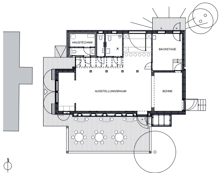
Grundriss Erdgeschoss, ohne Maßstab, Quelle: © Nalbach + Nalbach Gesellschaft von Architekten mbH, Berlin
